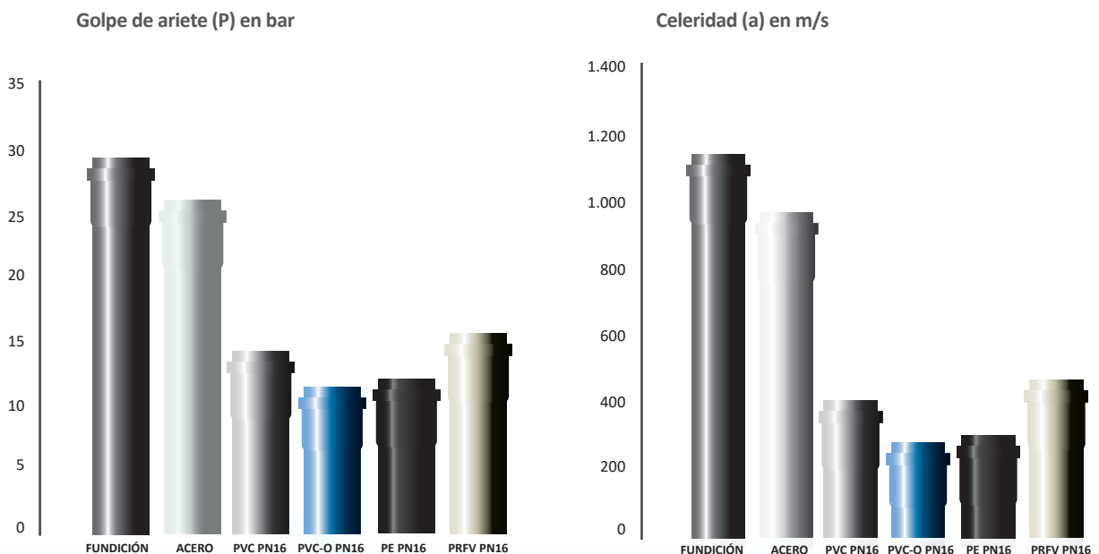
Sobrepresión producida al cerrar bruscamente una conducción con agua a 2,5 m/s.
