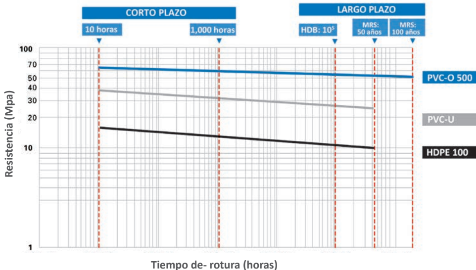
CURVA DE REGRESIÓN DE RESISTENCIA HIDROSTÁTICA
