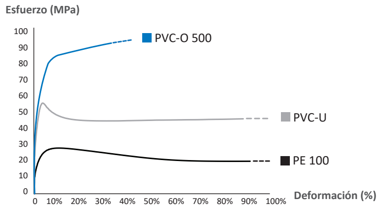
CURVAS DE ESFUERZO-DEFORMACIÓN
